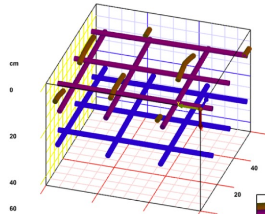
Vue 3D en perspective des deux lits d'aciers
