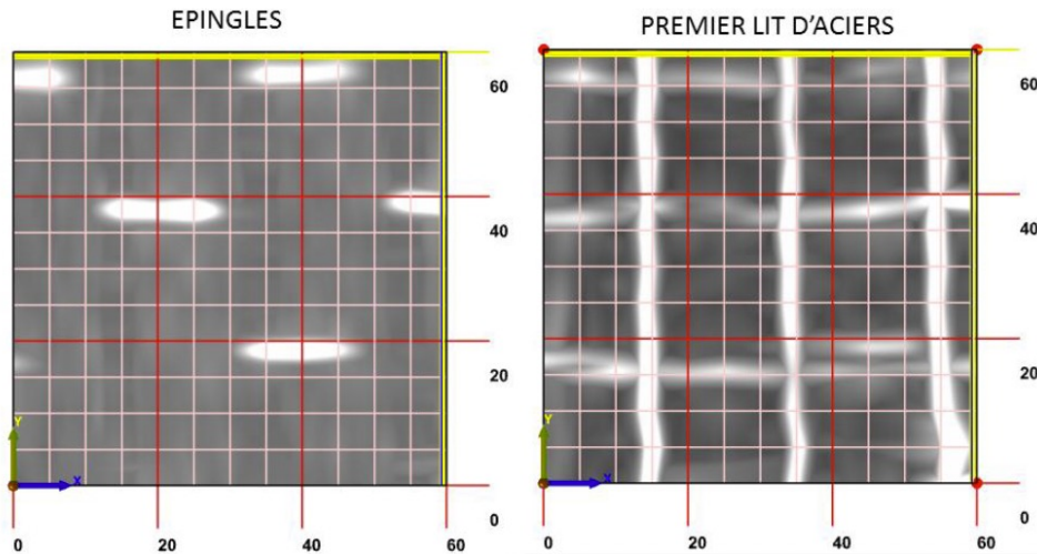
Grille 60x60cm 26 profils radar
