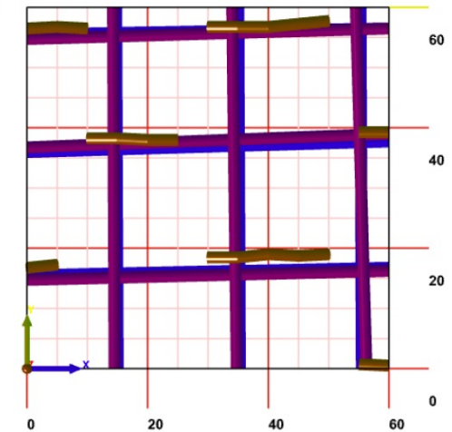
Vue 3D du dessus des deux lits d'aciers
