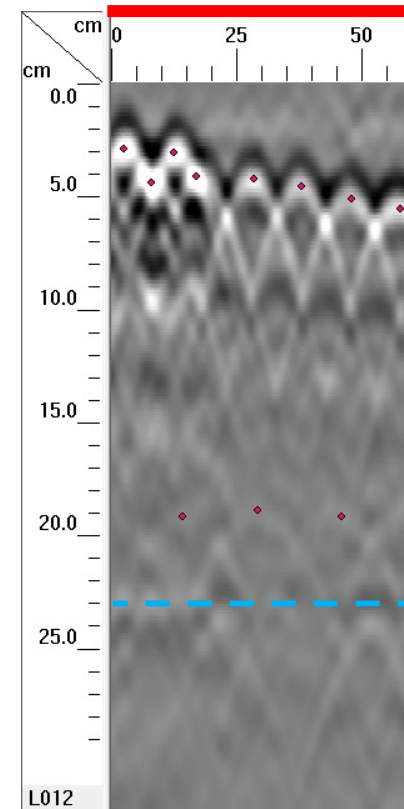
Vue en coupe Distance-Profondeur (B-SCAN)
